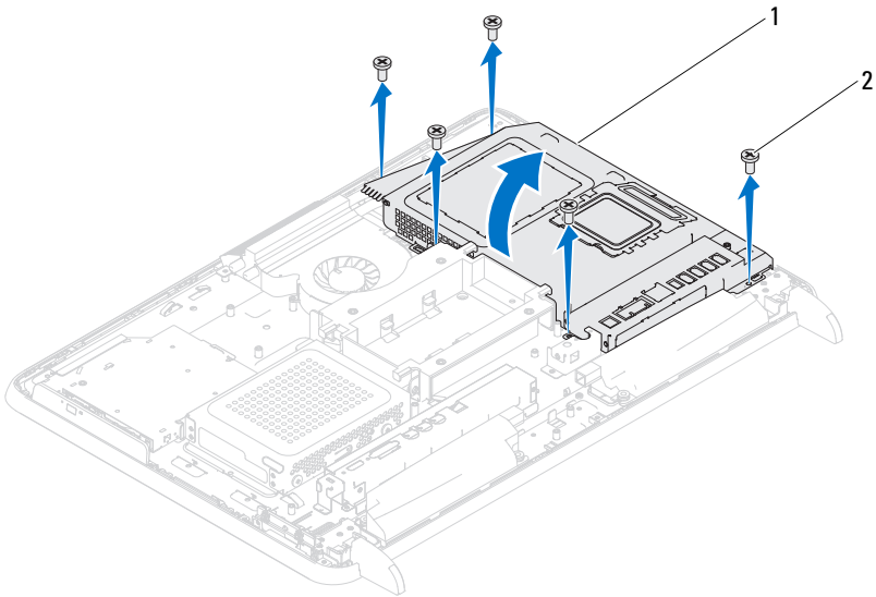
1 emolevyn suojus 2 ruuvit (5)
