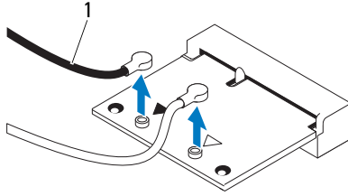
1 antennijohdot (2)
