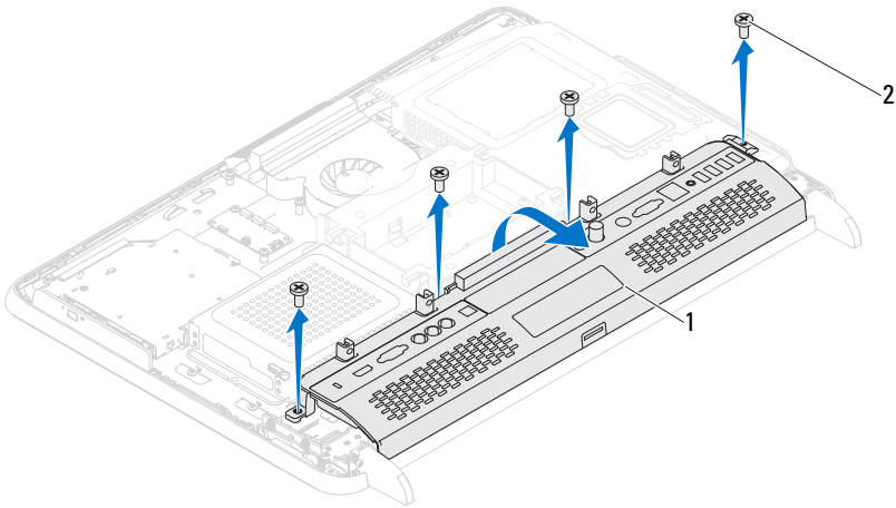
1 I/O-takasuojus 2 ruuvit (4)
