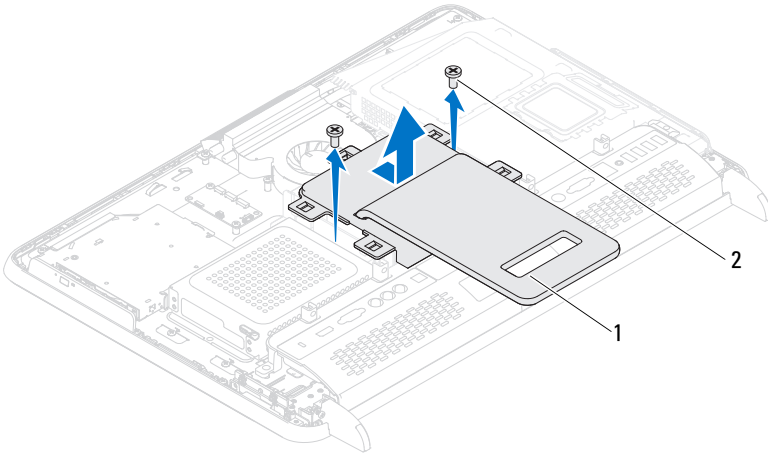
1 takatuen kokoonpano 2 ruuvit (2)
