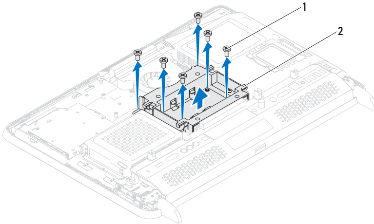
1 ruuvit (6) 2 VESA-teline
